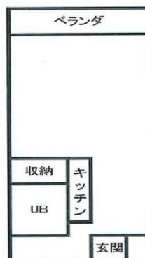
【平面図】
